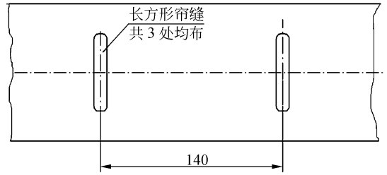
图 5 快门帘缝示意图
