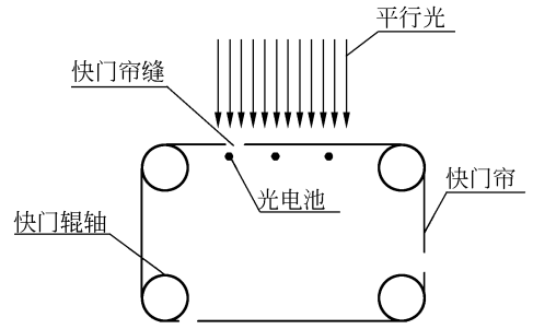
图 7 快门曝光时间及快门帘运动速度均匀性检测原理
