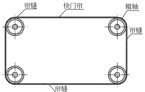
图 3 环形帘的焦面帘幕式快门帘形式示意图
