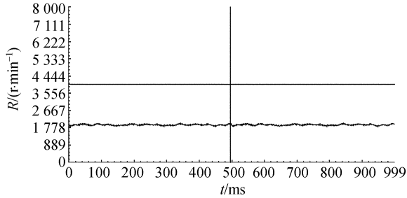
图 6 电机转速测试结果
