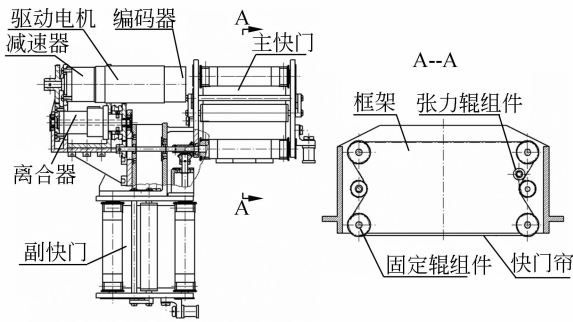
图 4 快门组件结构简图
